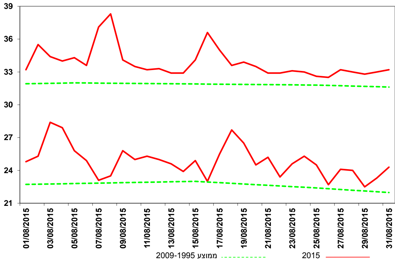
איור 2: טמפרטורת המינימום והמקסימום היומית בבית דגן באוגוסט 2015 לעומת הממוצע הרב שנתי
